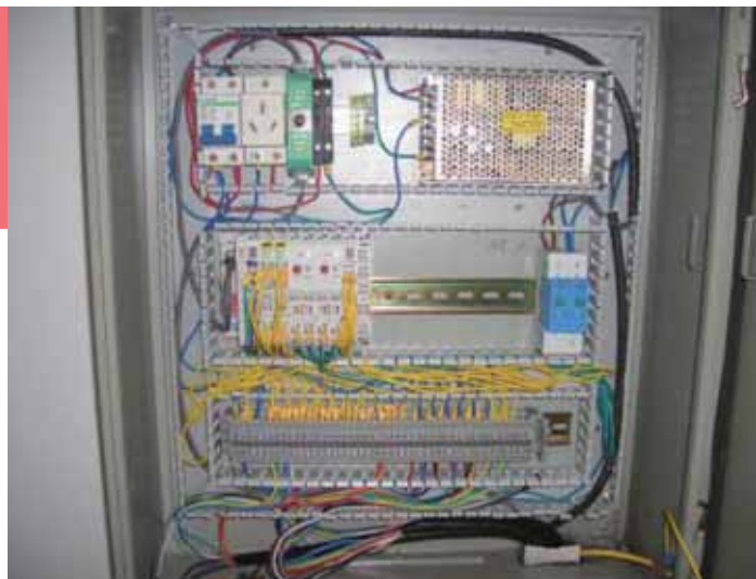
配电箱内布置
