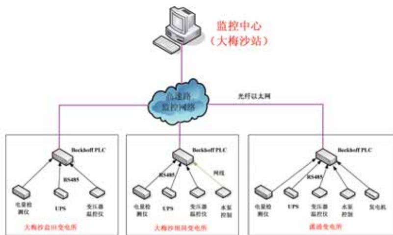
网络结构图
