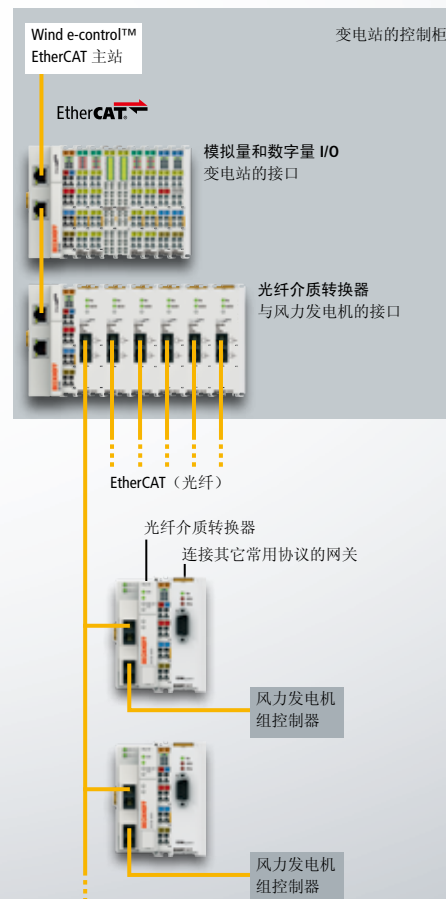
EtherCAT 拓扑结构的整体示意图显示风场中由各个具体模块处理的功能
