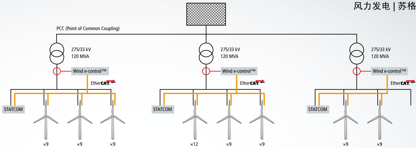
Wind e-control™ 系统用于每个变电站，确保风场中各个风力发电机之间的 EtherCAT 数据传输安全
